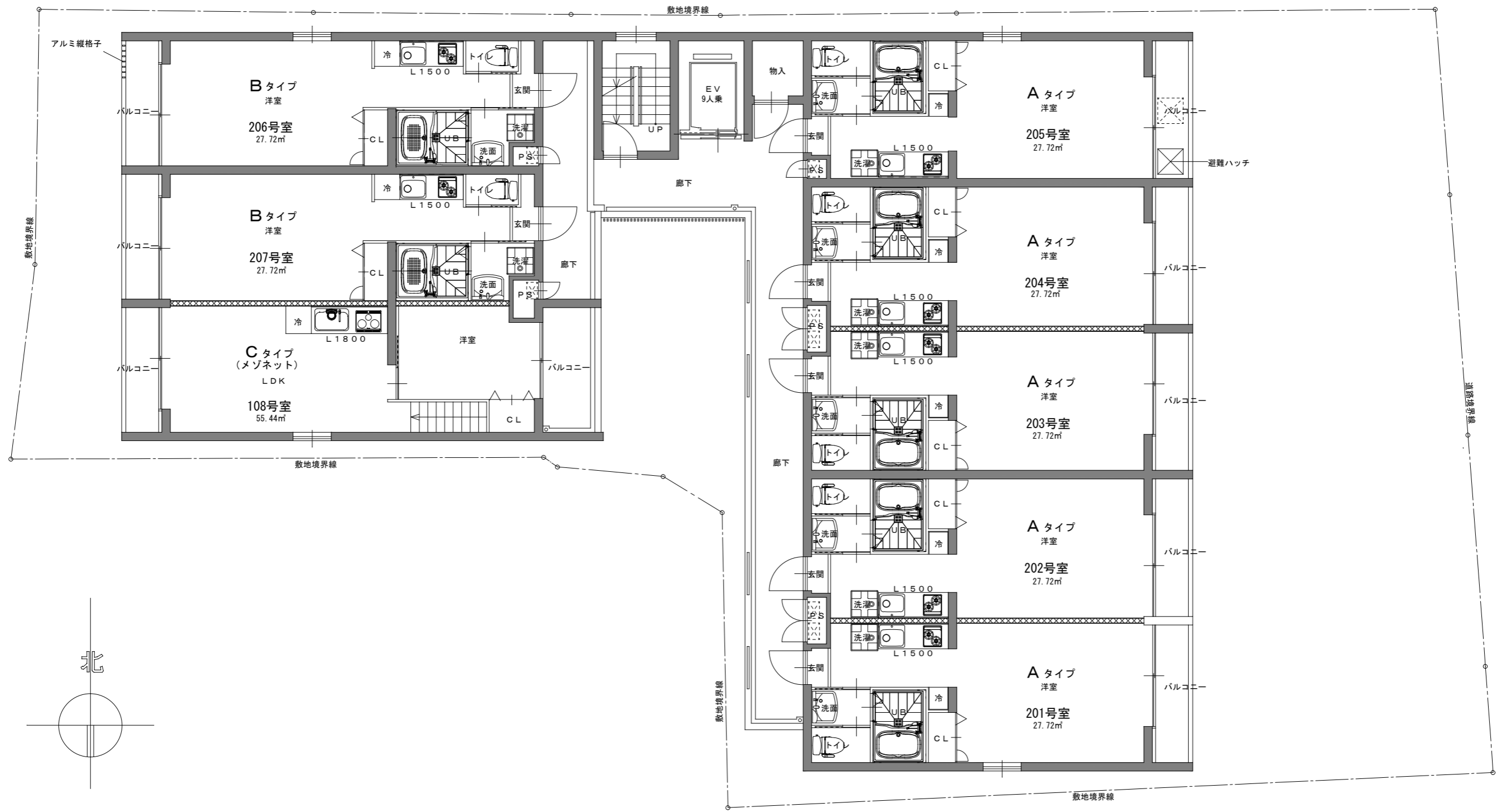
2階平面図
