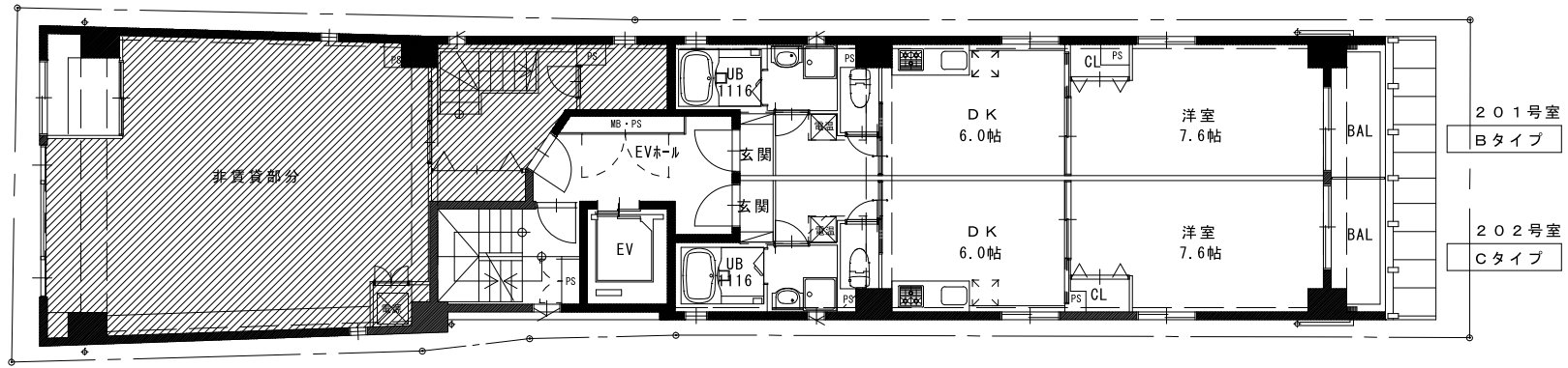
2階平面図
