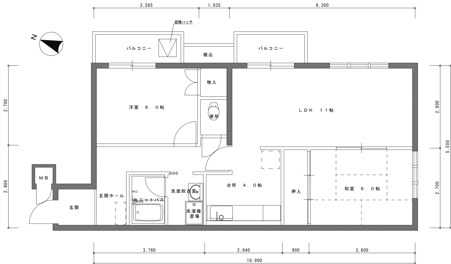
B2 TYPE 平面図
