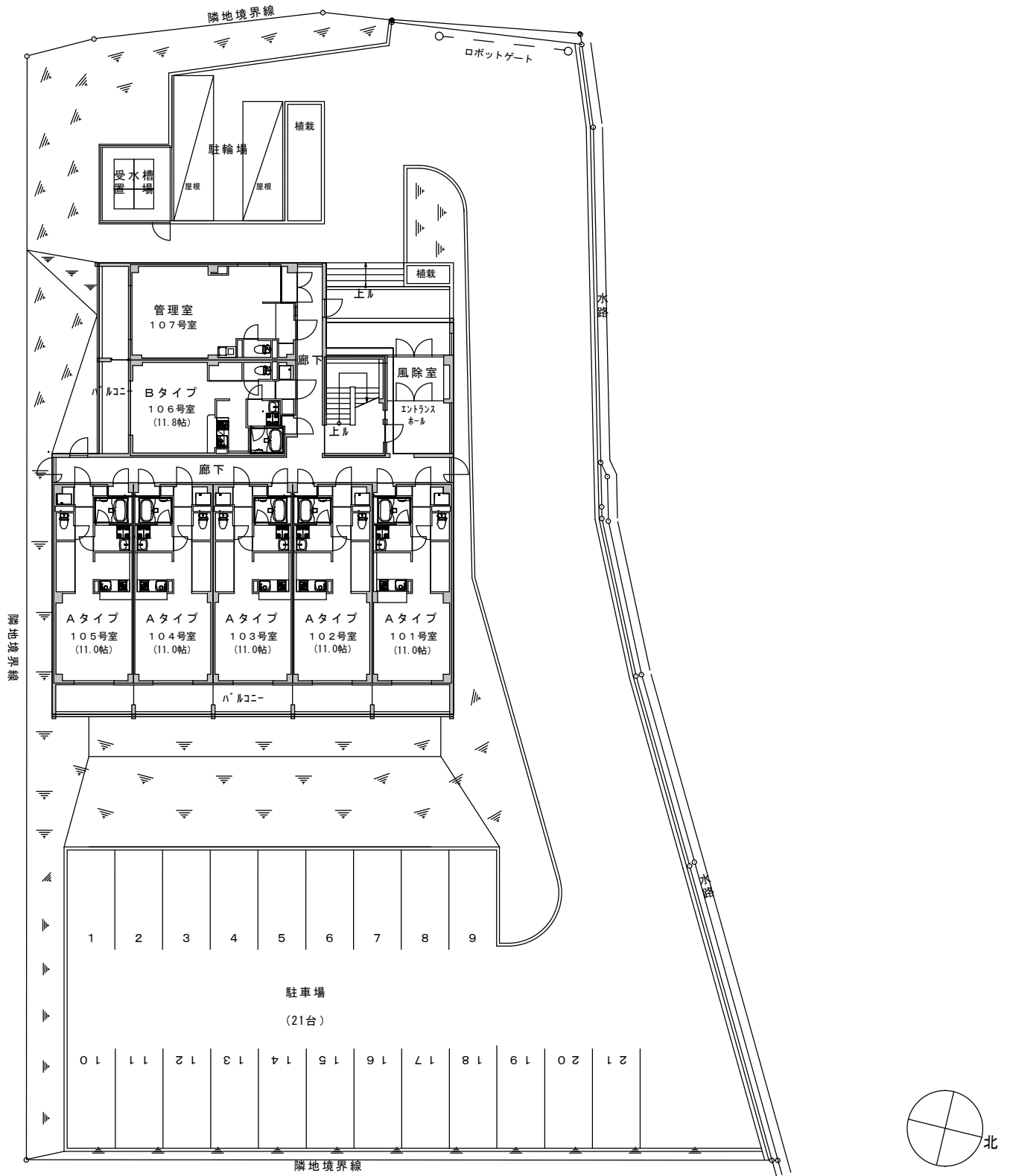
配置図
