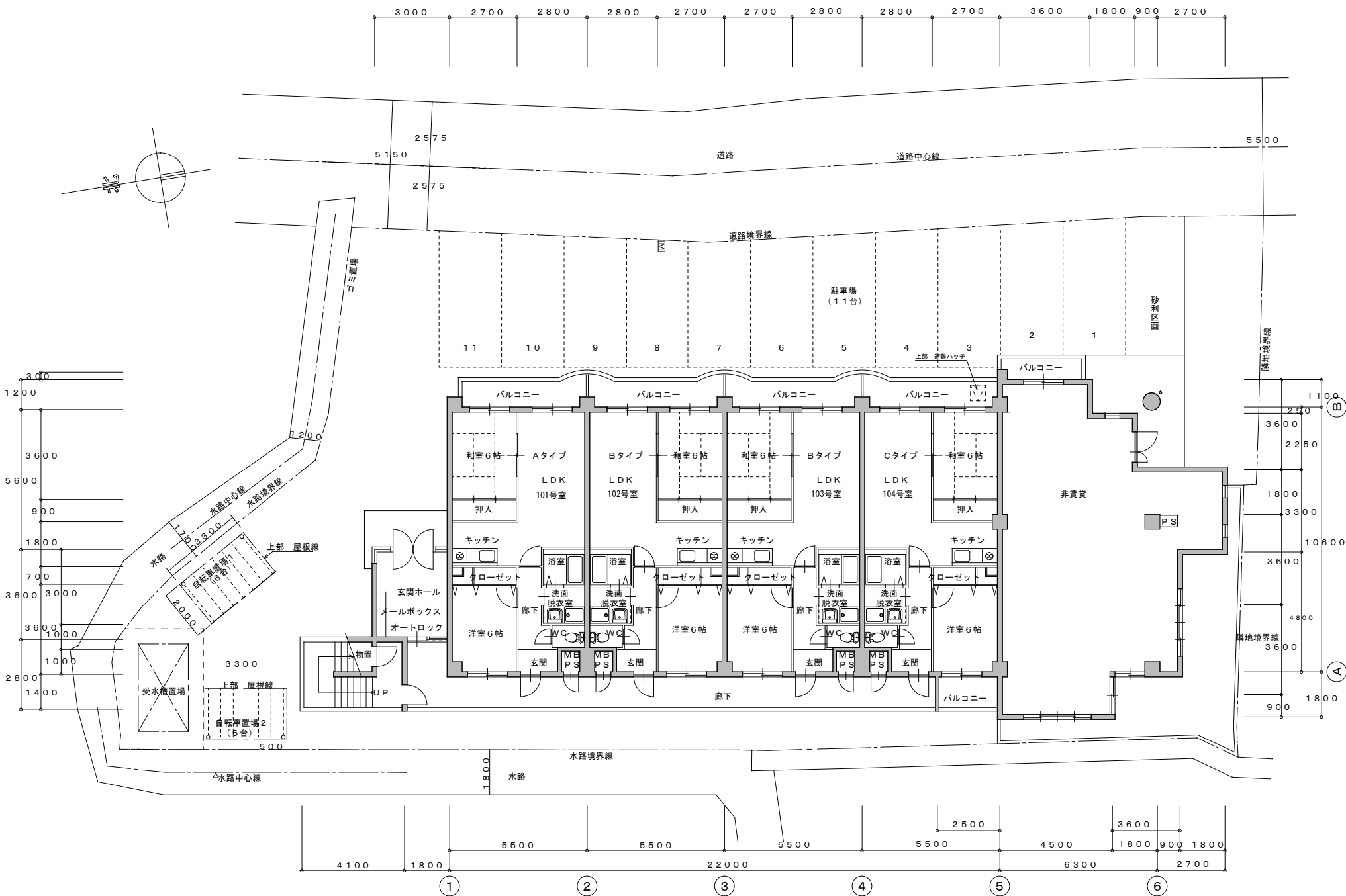
1階平面図
