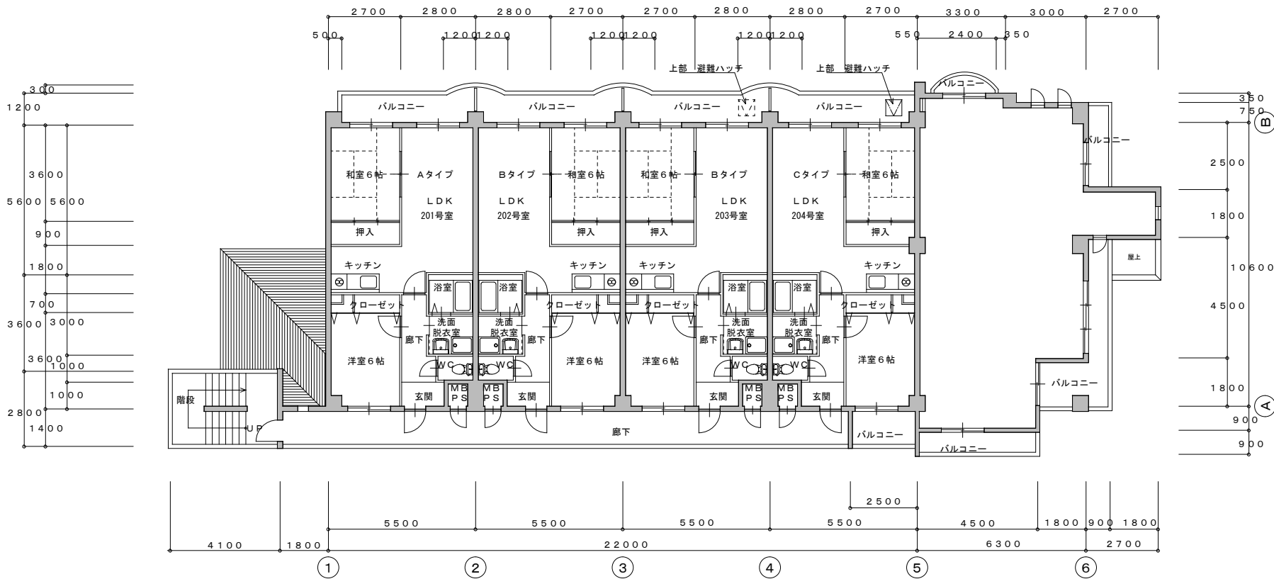
2階平面図
