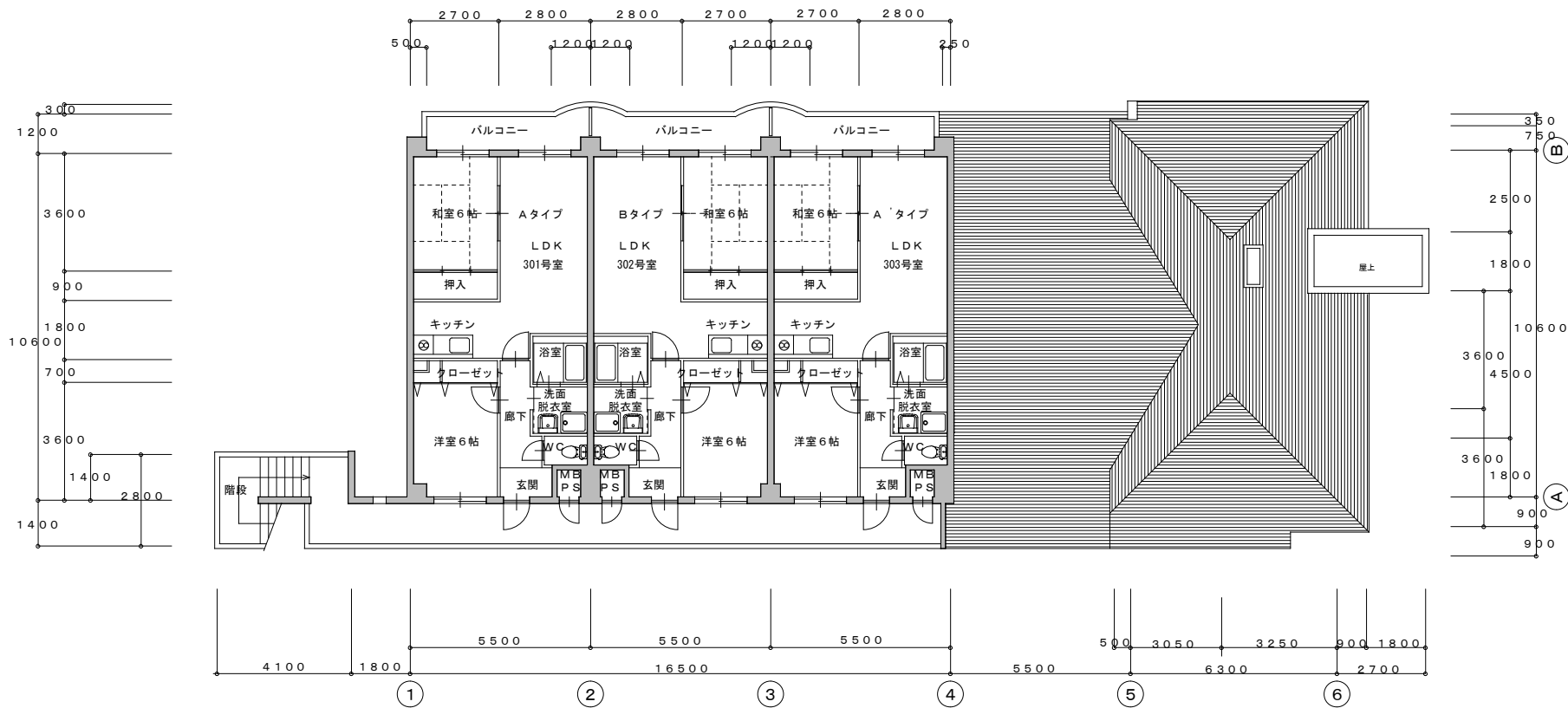
3階平面図
