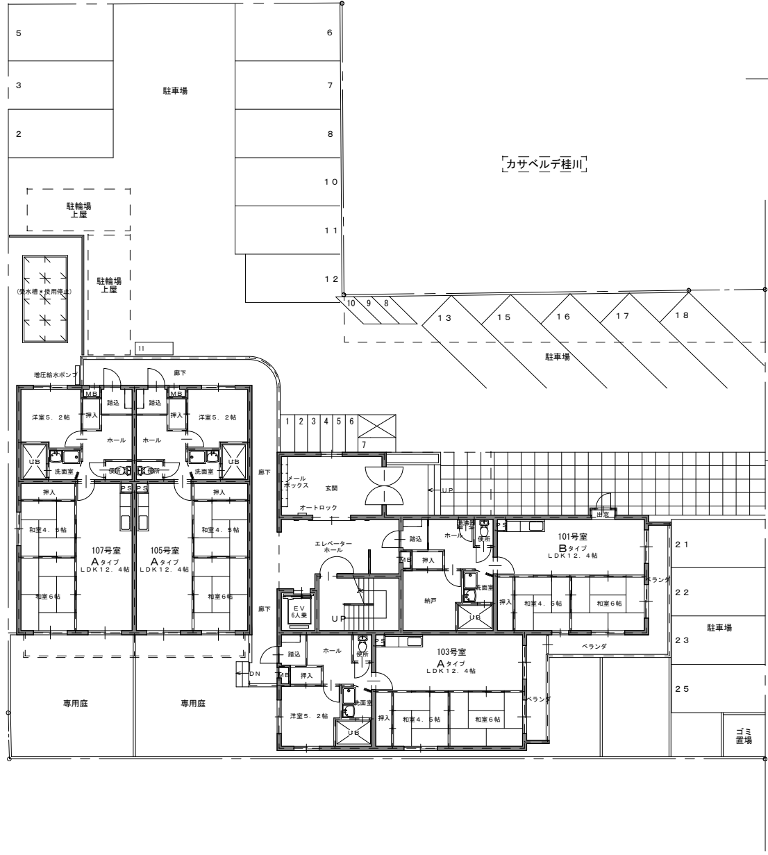
配置図・1階平面図
