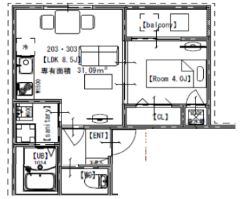
03号室(31.09 ㎡)
