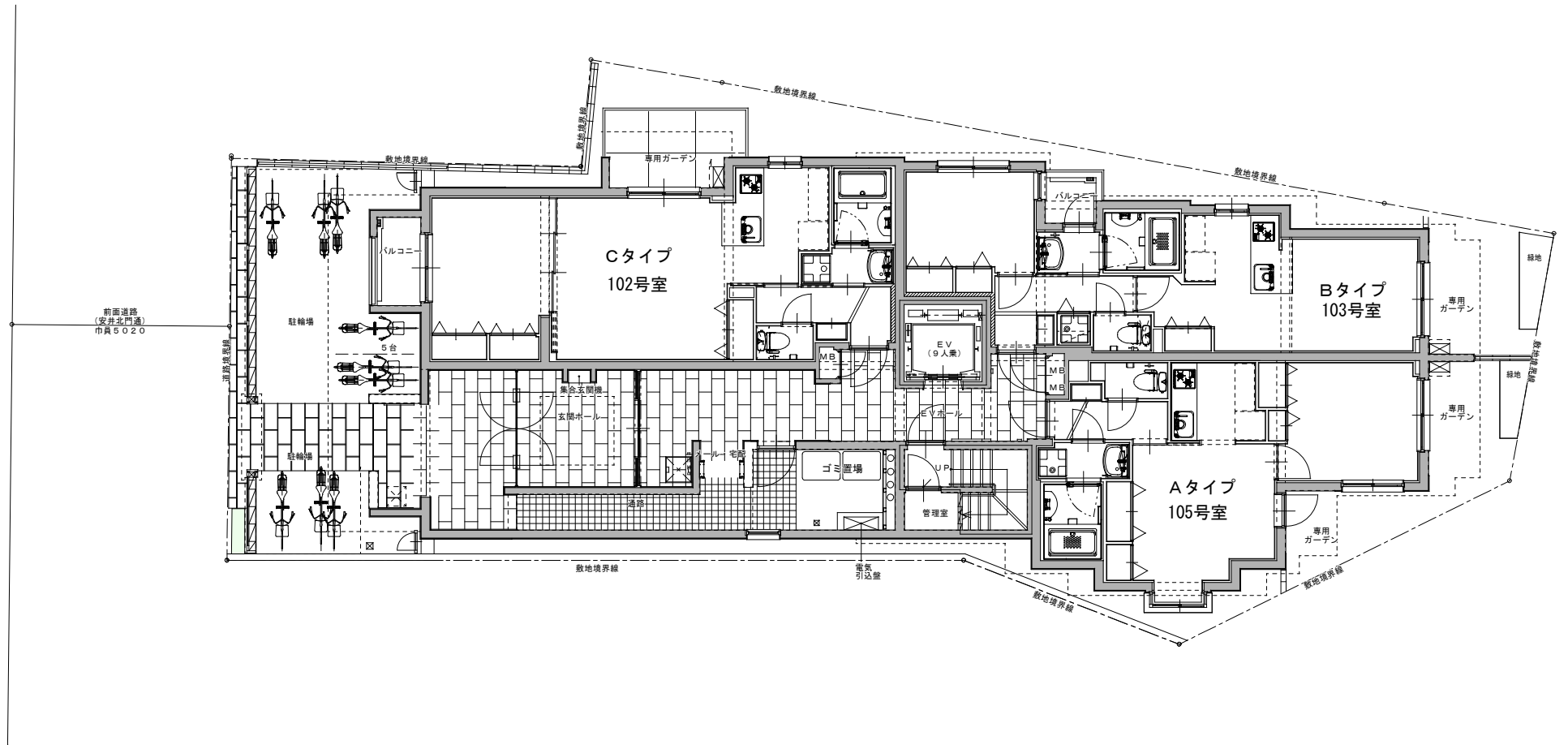
1階平面図
