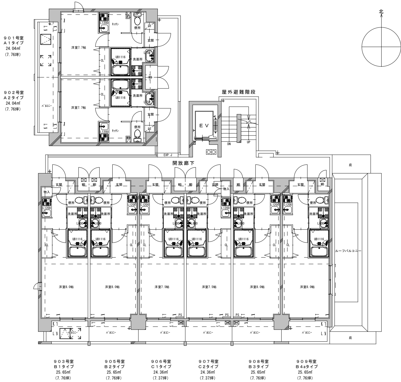
9階平面図
