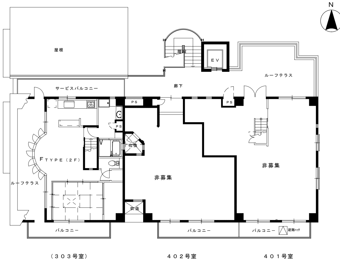
4階平面図
