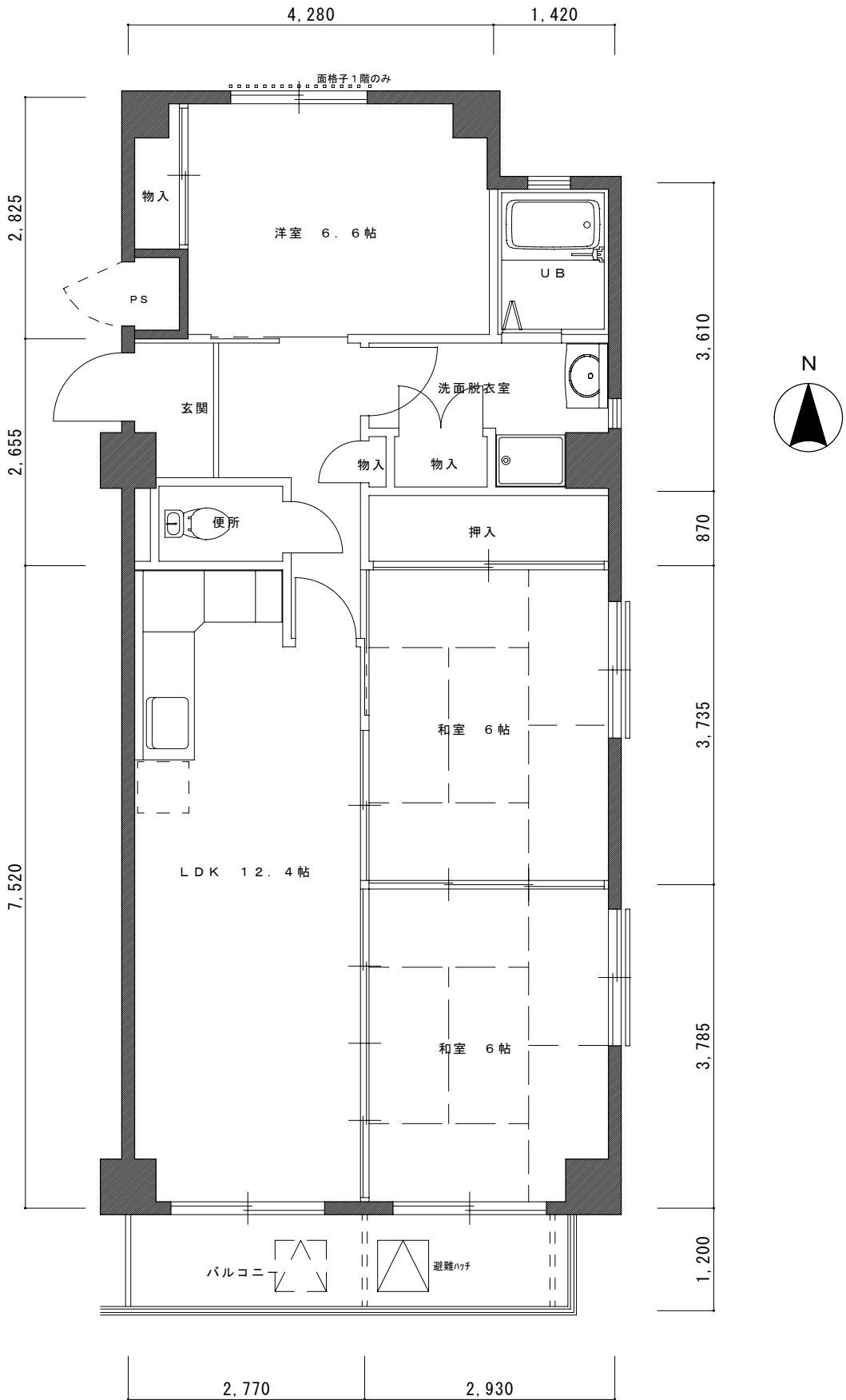
A TYPE 平面図
