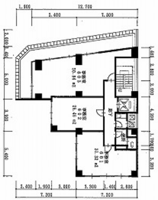
6階 平面図
