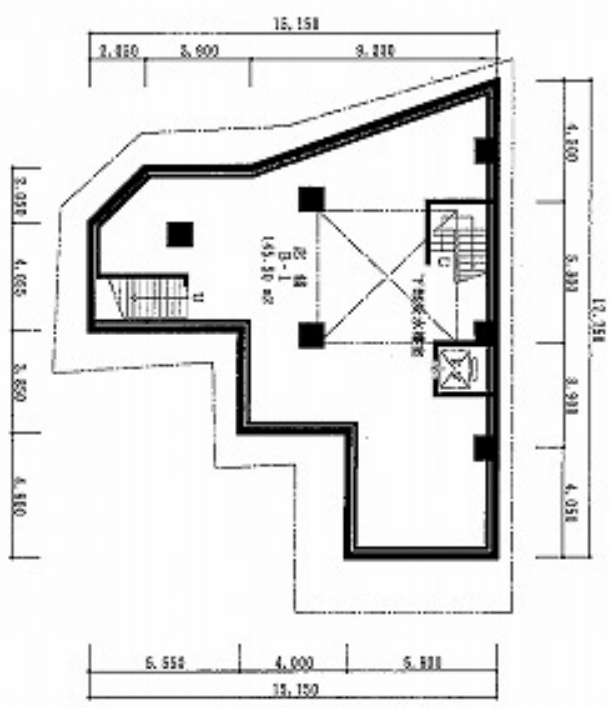
地下1階 平面図
