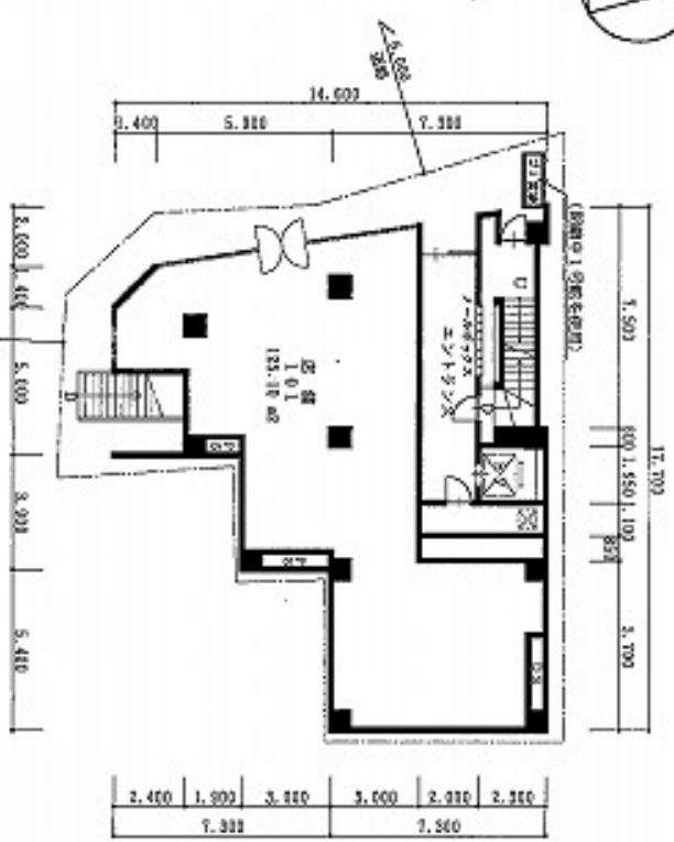
1階 平面図
