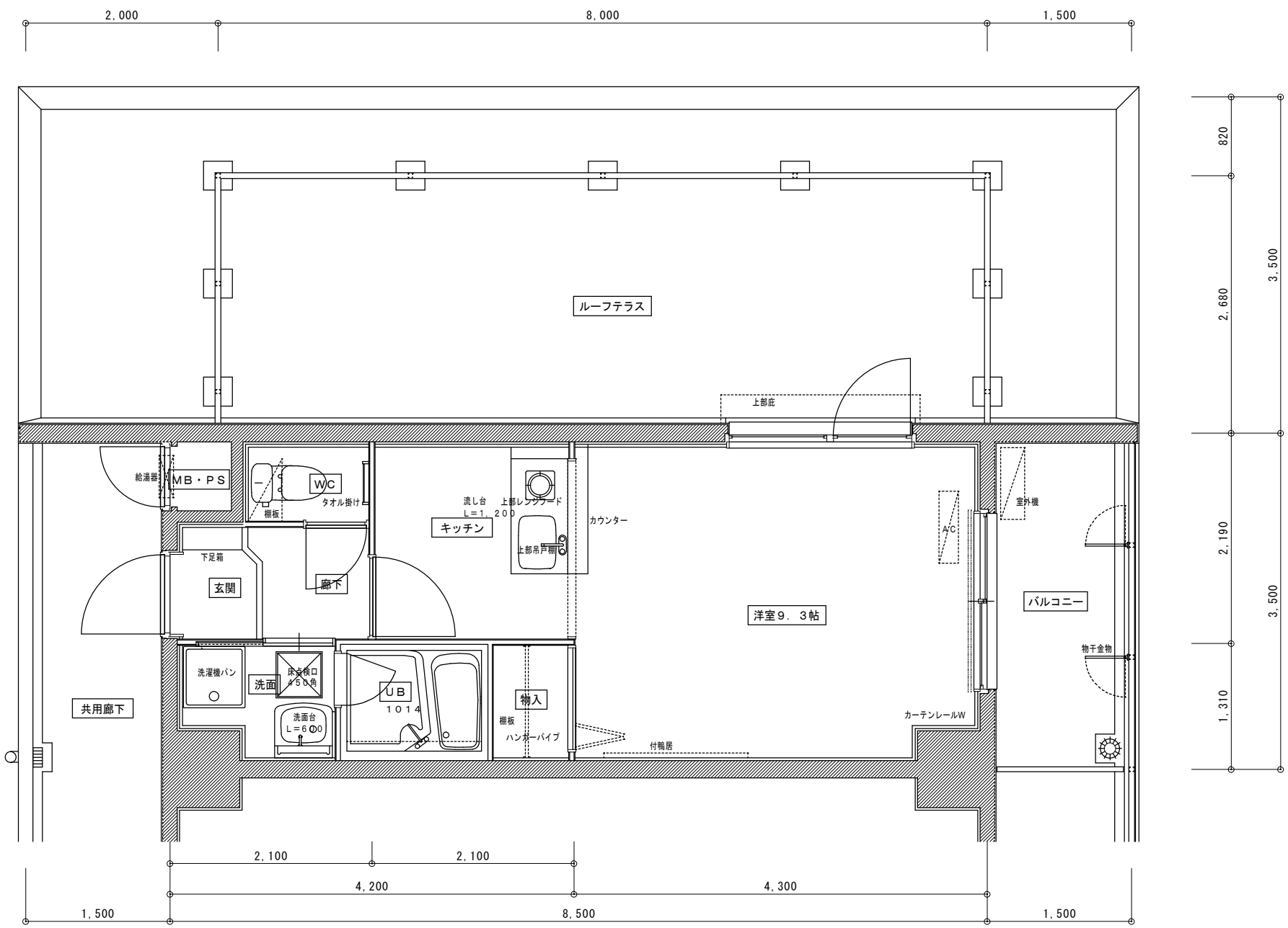
601号室 Aタイプ平面詳細図 (ルーフテラス付き)
