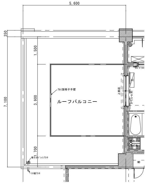
6階平面詳細図
