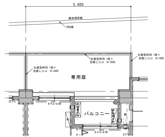
専用庭平面詳細図
