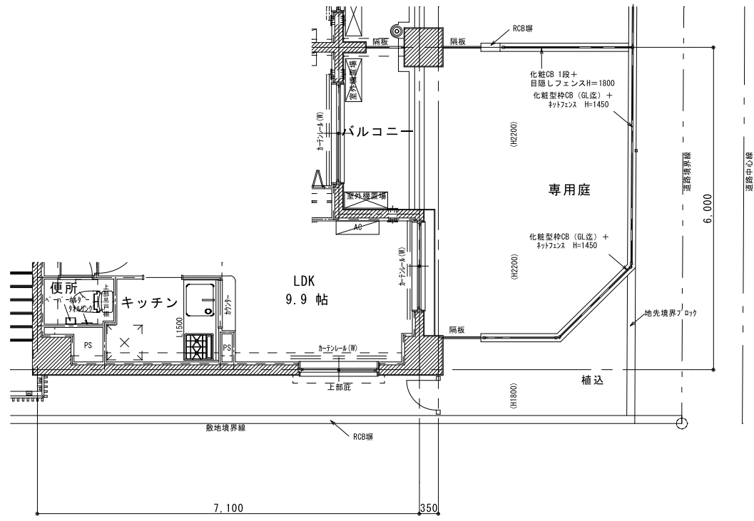
専用庭平面詳細図
