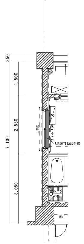
7階平面詳細図
