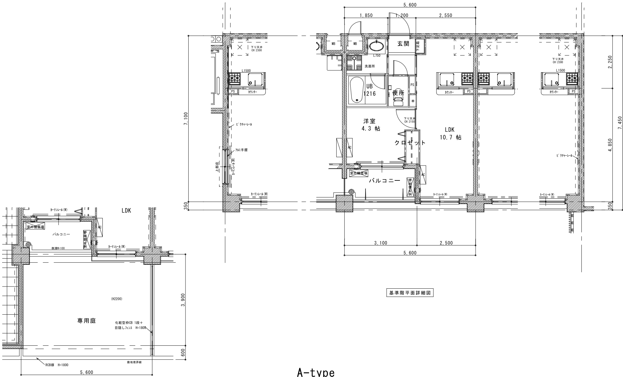
専用庭平面詳細図
