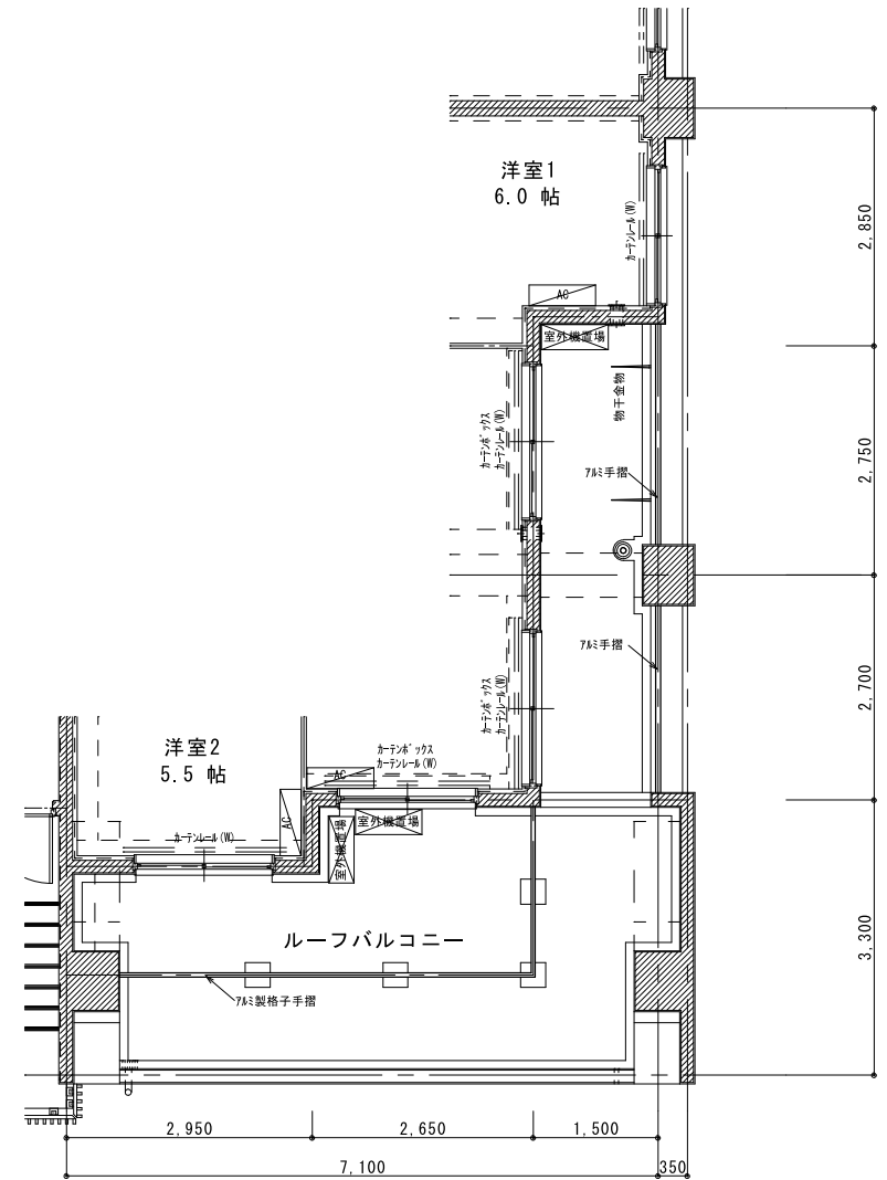
4階平面詳細図
