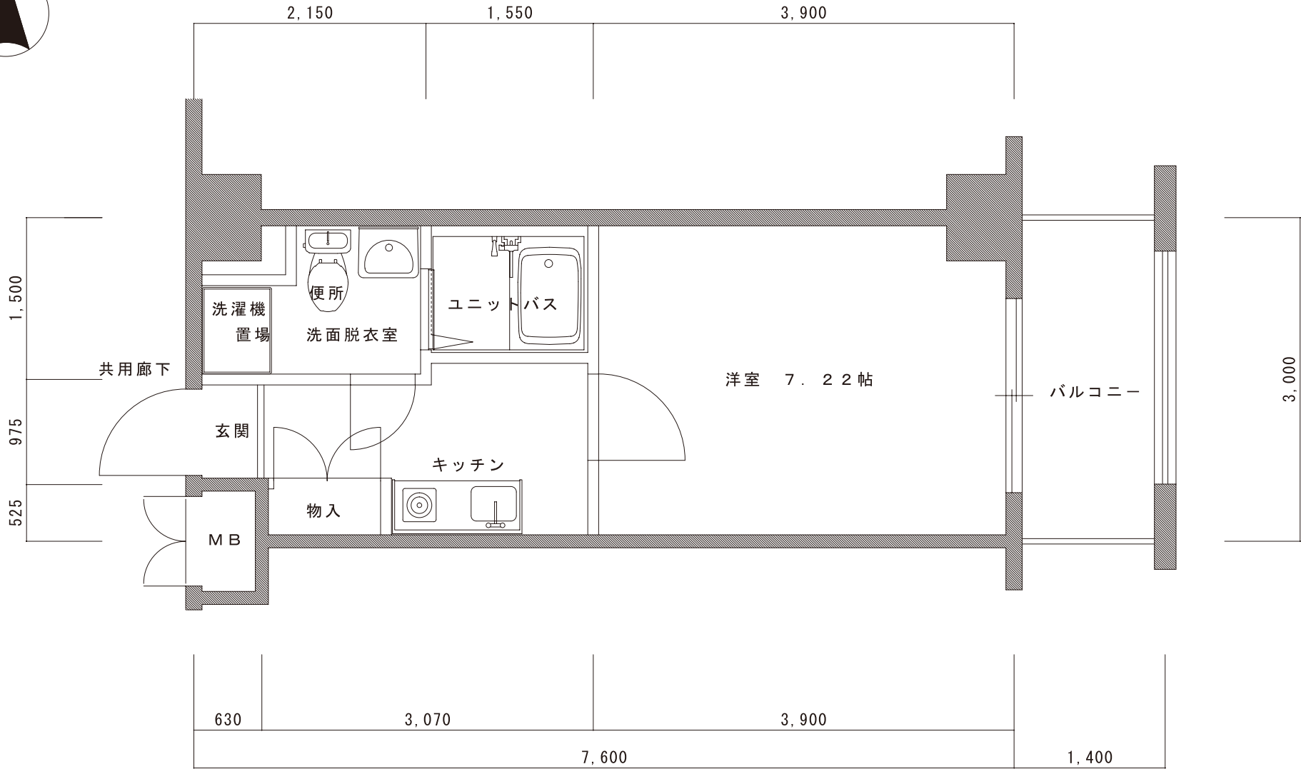
A TYPE 平面図
