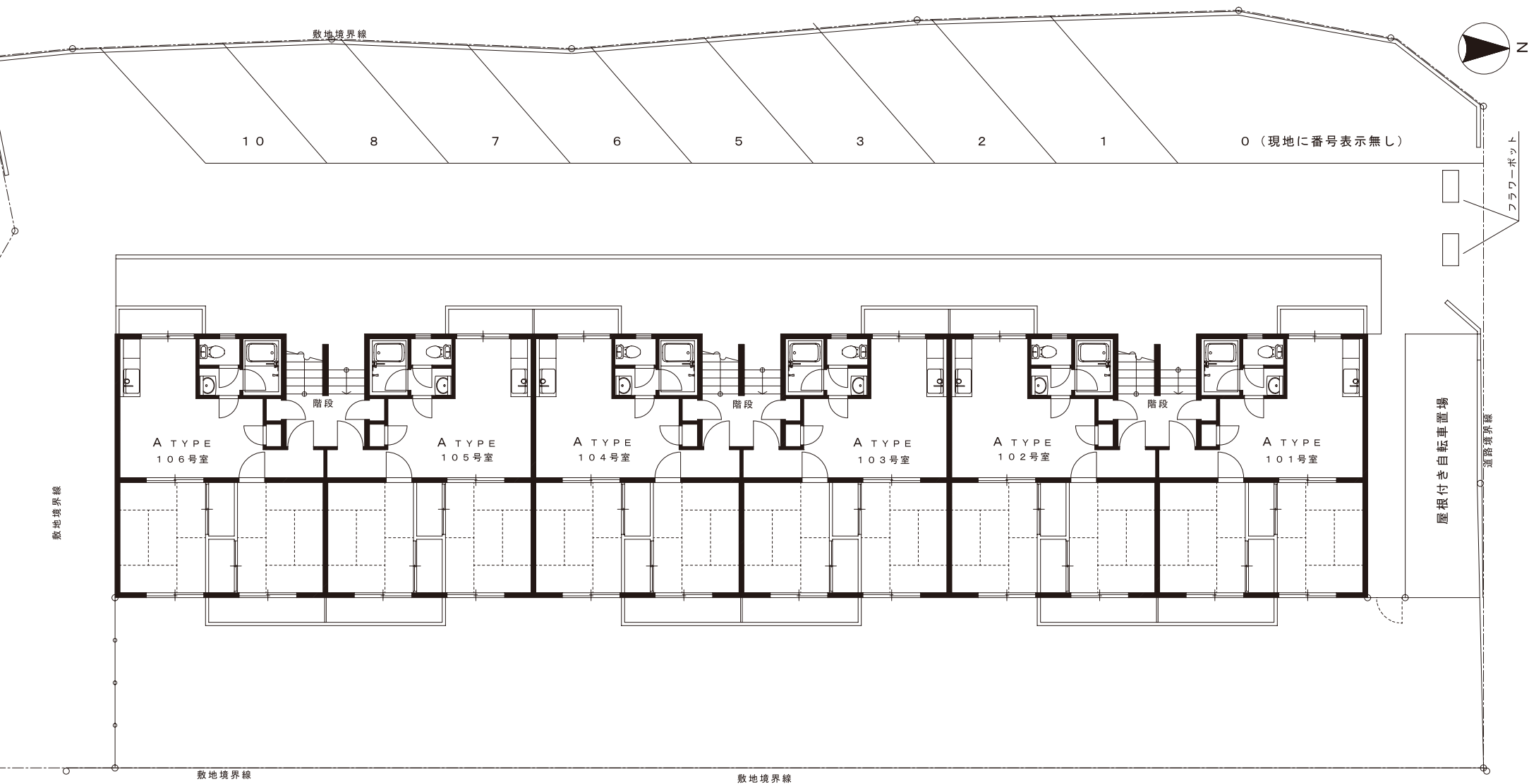
配置図 1階平面図
