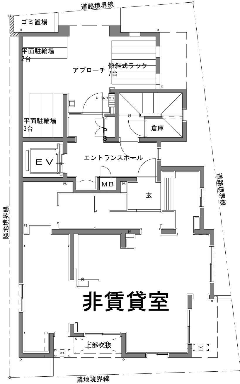
1 階平面図
