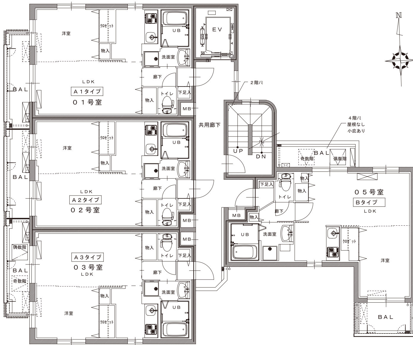
2～4階平面図
