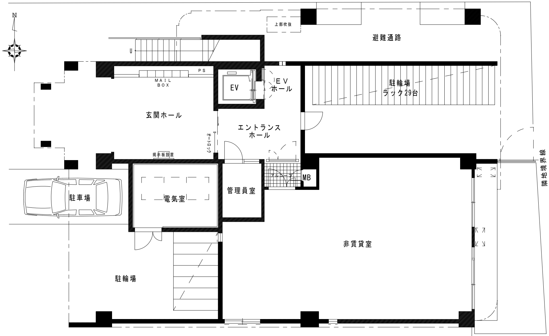
配置図
