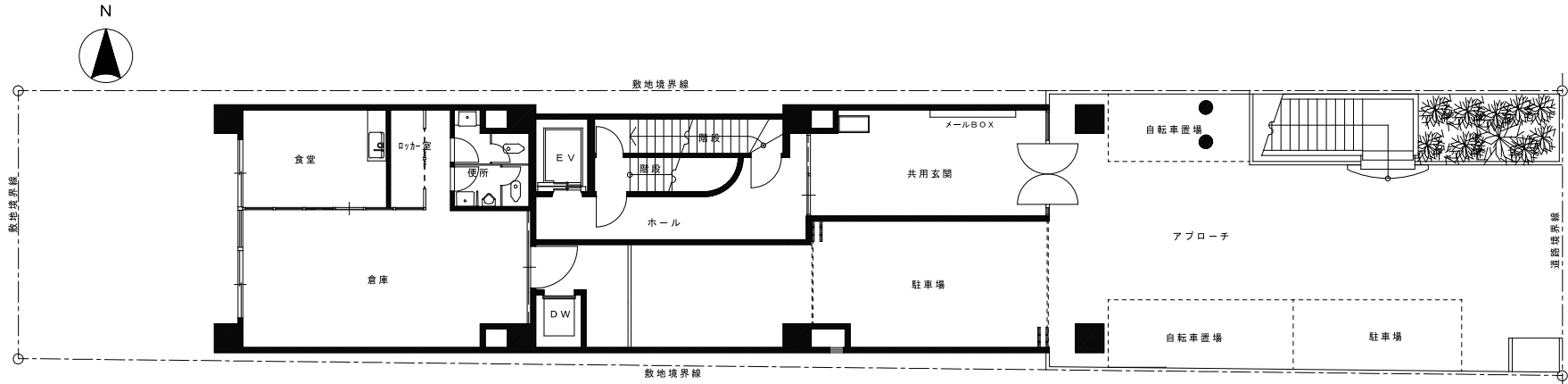
配置図 1階平面図
