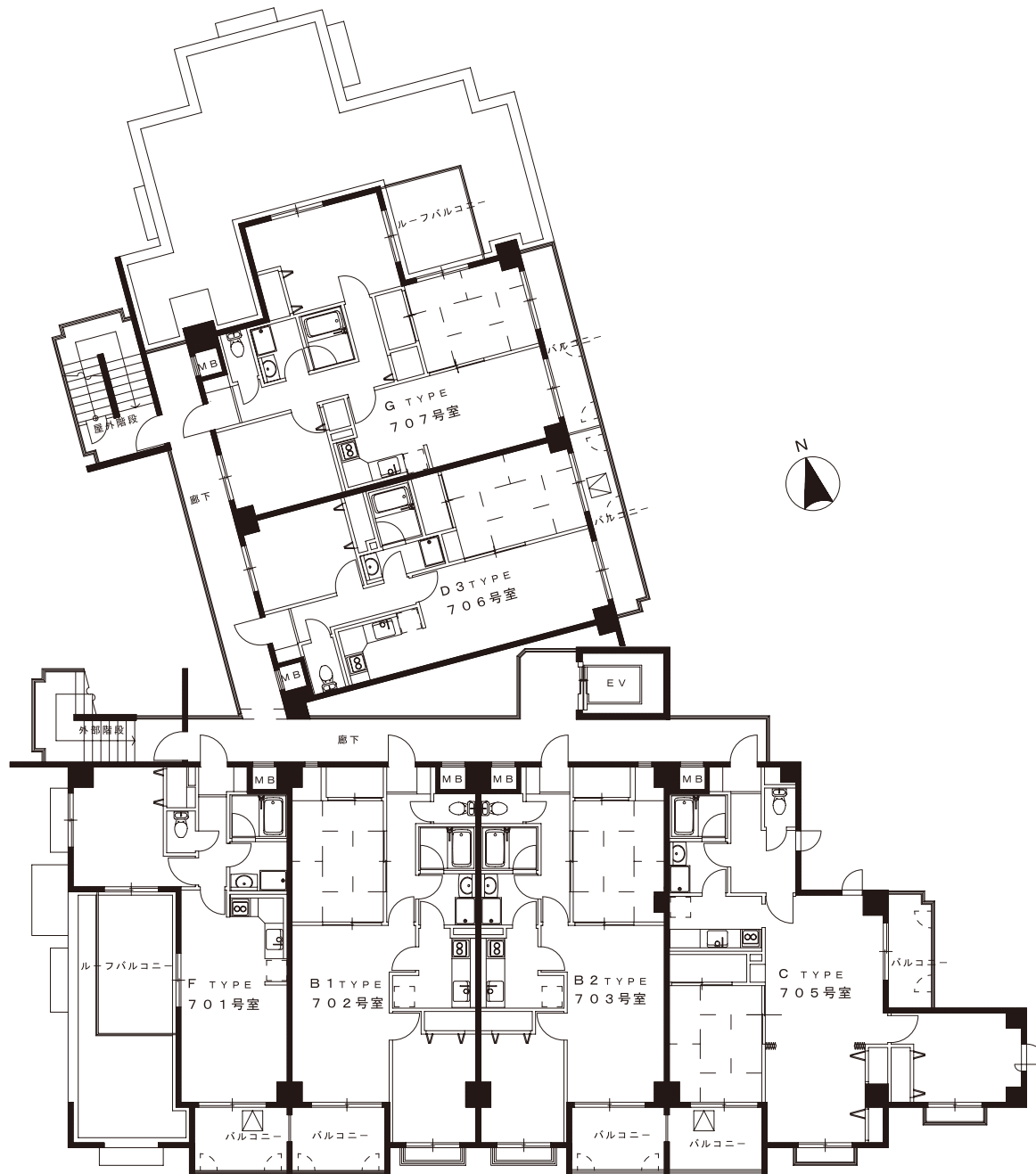
7階平面図
