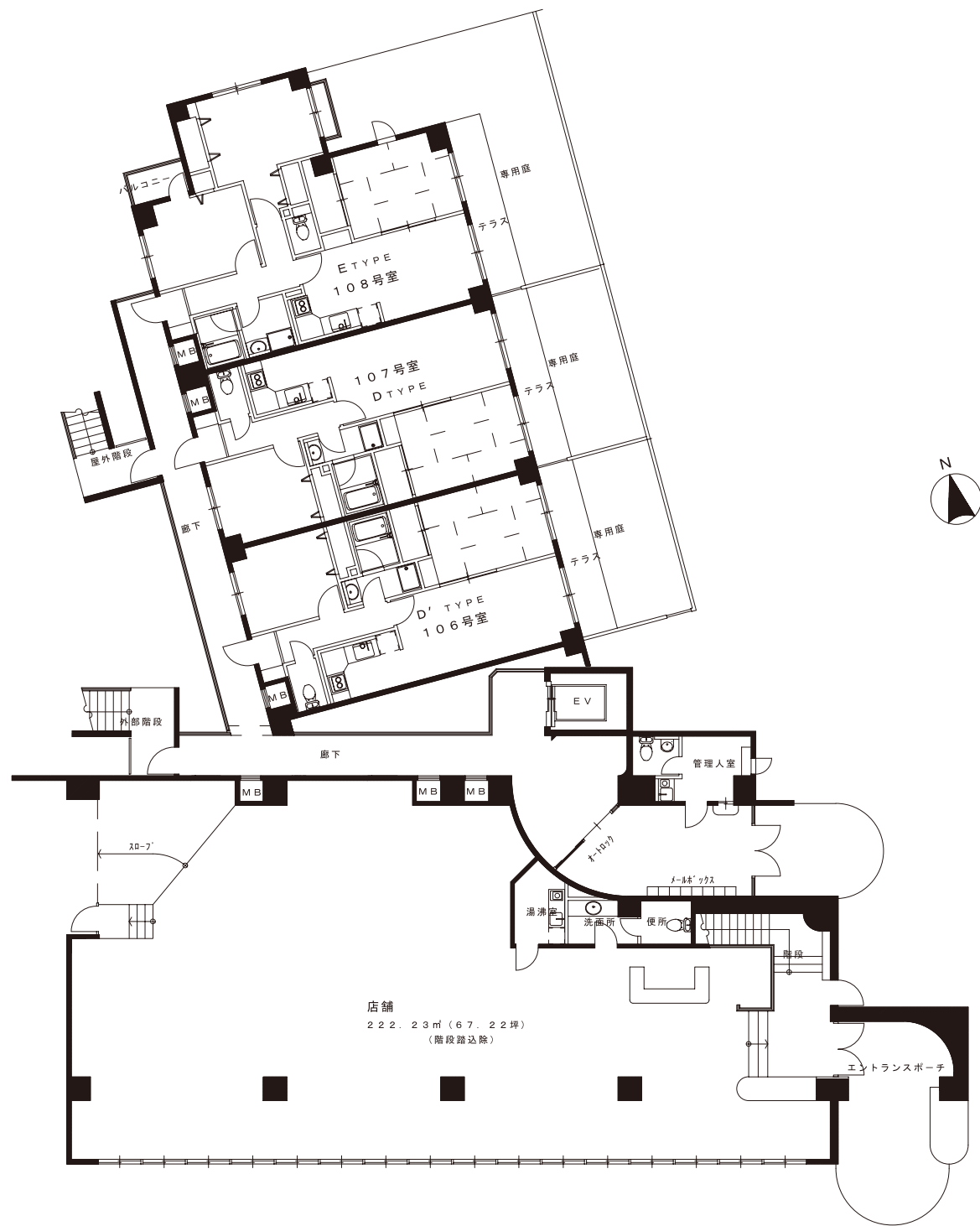
1階平面図
