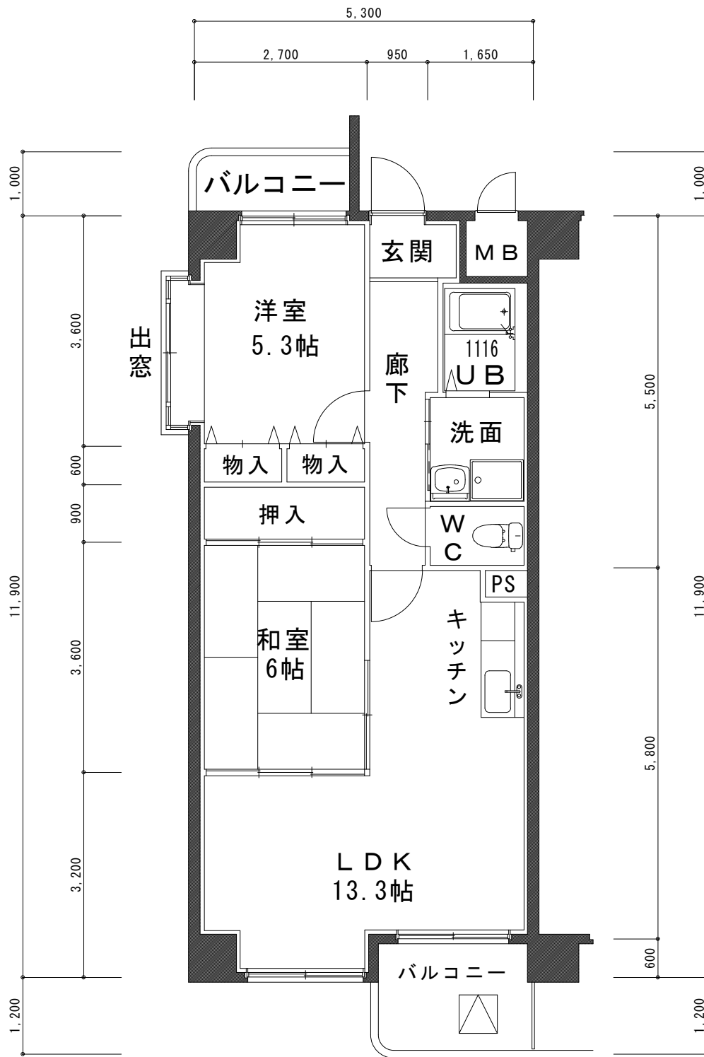
Aタイプ 60.47m 2
