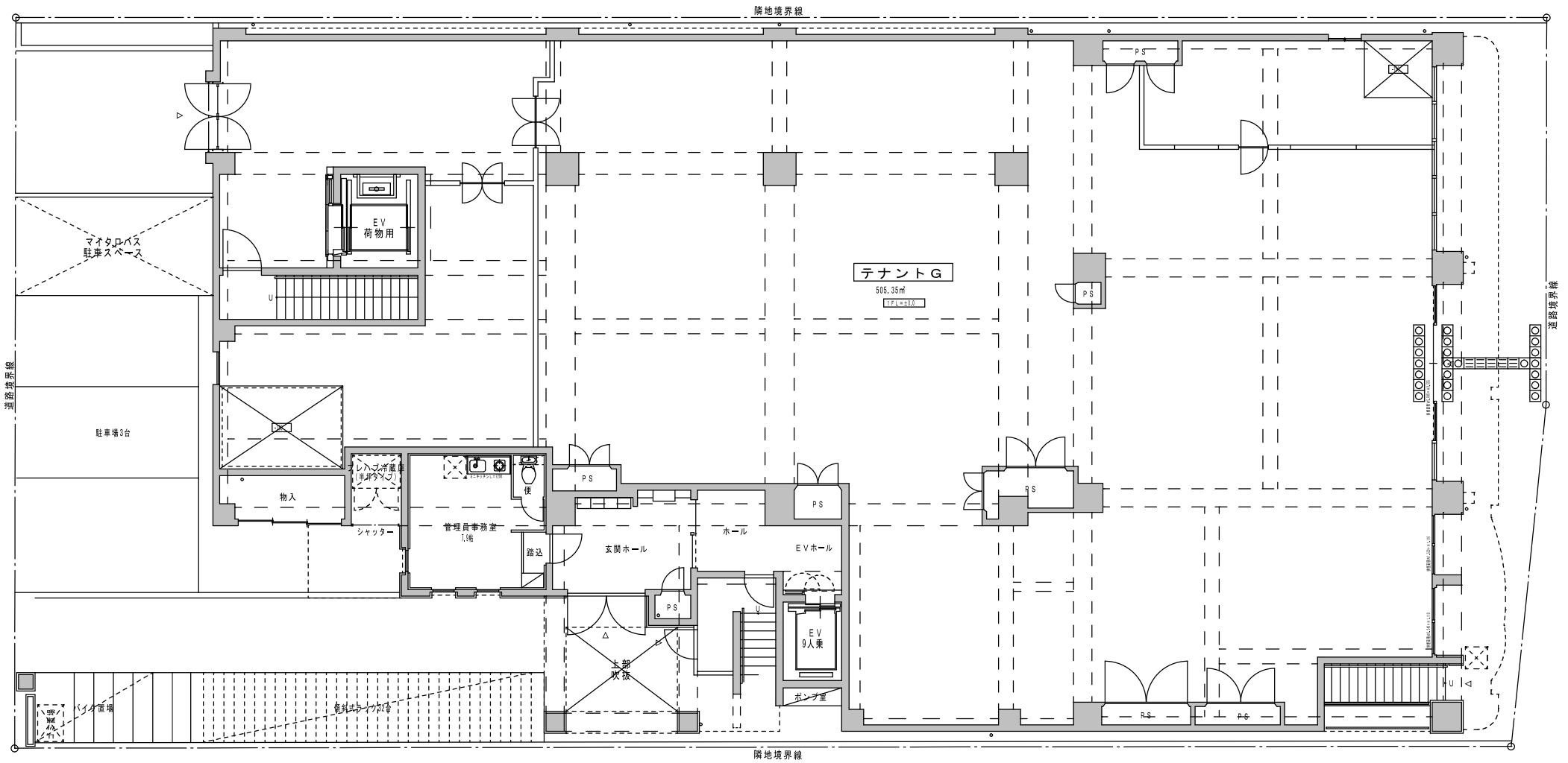
1階平面図
